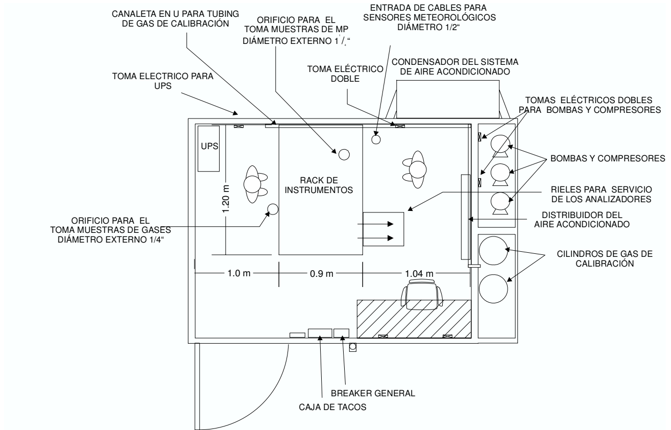
Figura 2-4. Ejemplo de distribución de equipos al interior de estación
