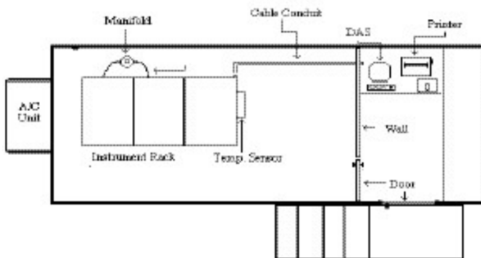
Figura 2-5. Otro ejemplo de distribución de equipos en la estación (EPA)
