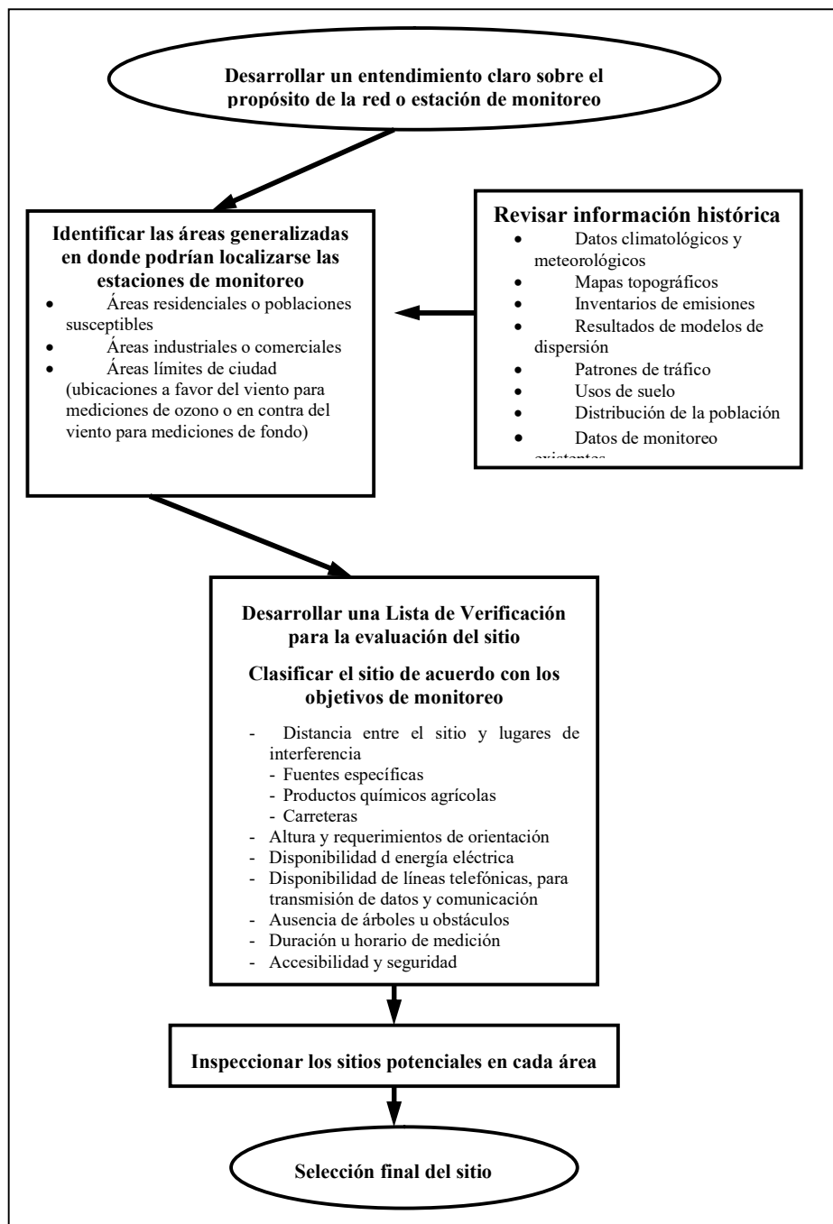
Figura 2-2. Esquema general de selección del sitio
