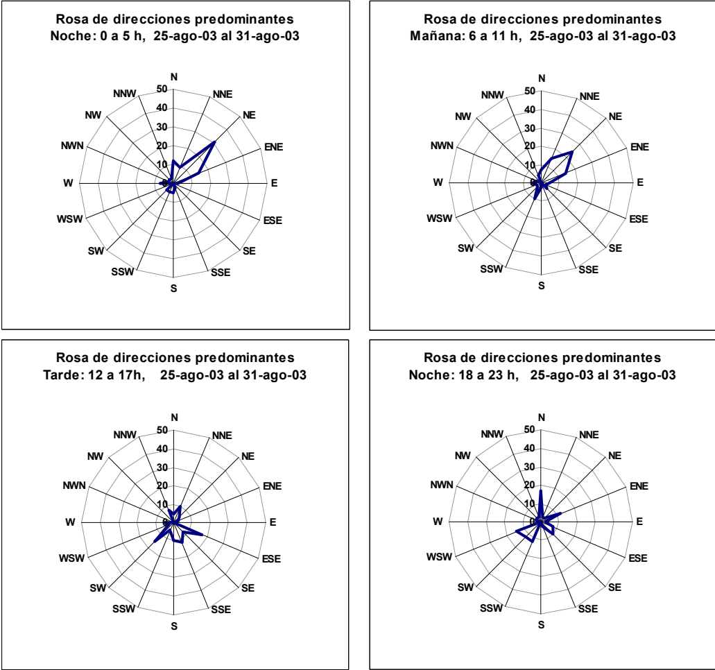
Figura 8: Rosas de direcciones de viento predominantes
