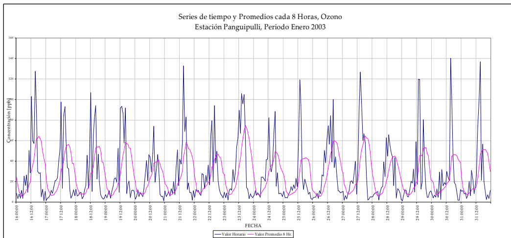
Figura 6-4 Ejemplo reporte mensual de mediciones continuas de gases (continuación)
