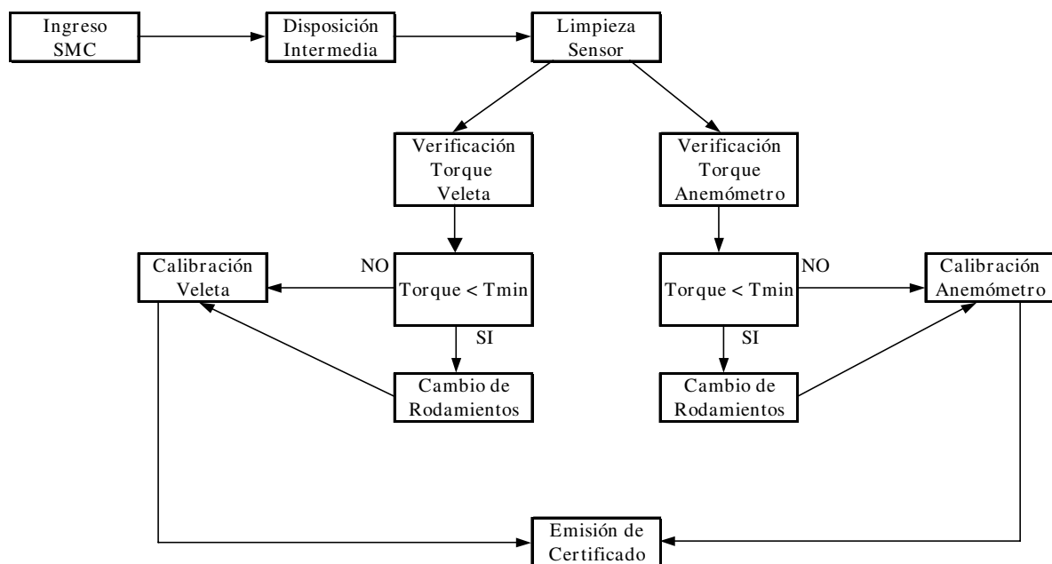
Figura 8.2 Línea de Calibración de sensores de Viento Tipo anemómetro integrado
